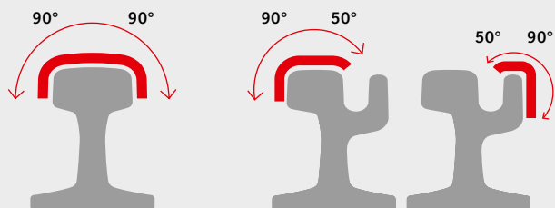
Obszar szlifowania
