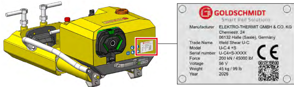
Abb. 2-4 Typenschild
