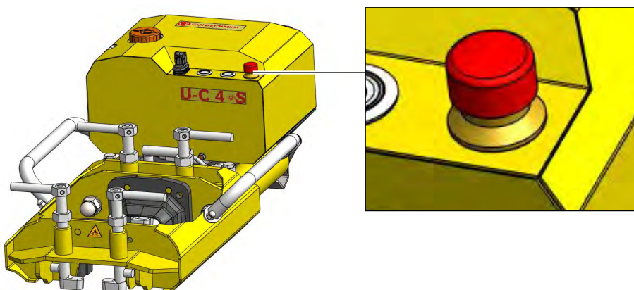
Abb. 2-7 Sicherheitseinrichtungen: Not-Halt-Taster
