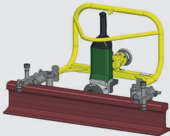
Amolado de la cara activa/borde de rodadura
