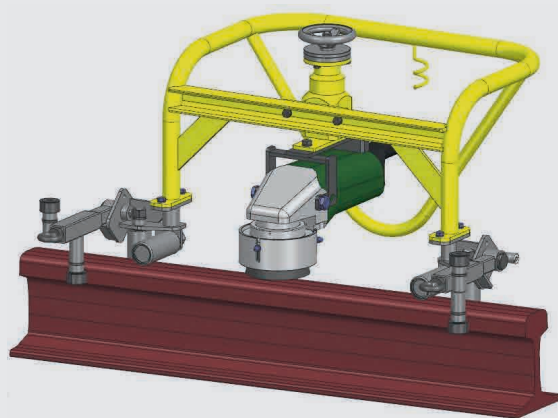
Amolado de la superficie de rodadura
